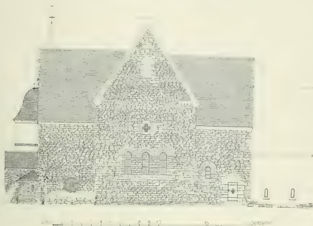
Fig. 18. Kyrkans östra fasad. Efter uppmätning av S. Curman o. A. Roland 1907, kompletterad av H. Sundberg 1927.
